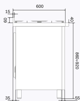
Vista laterale
